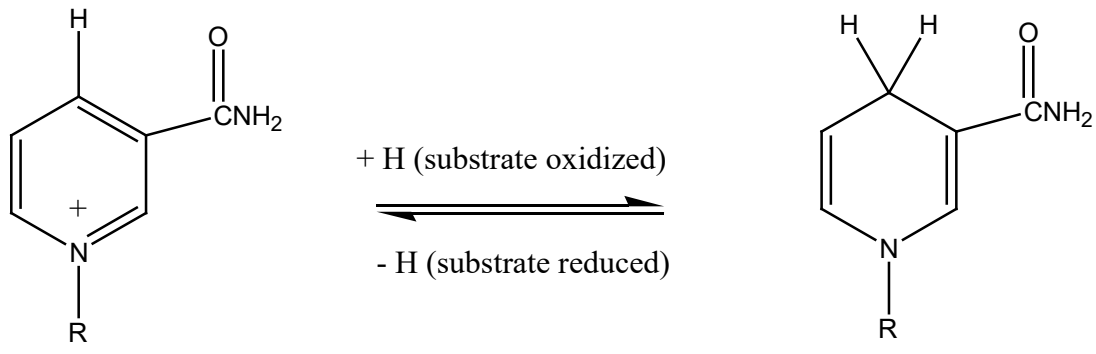
NAD +
